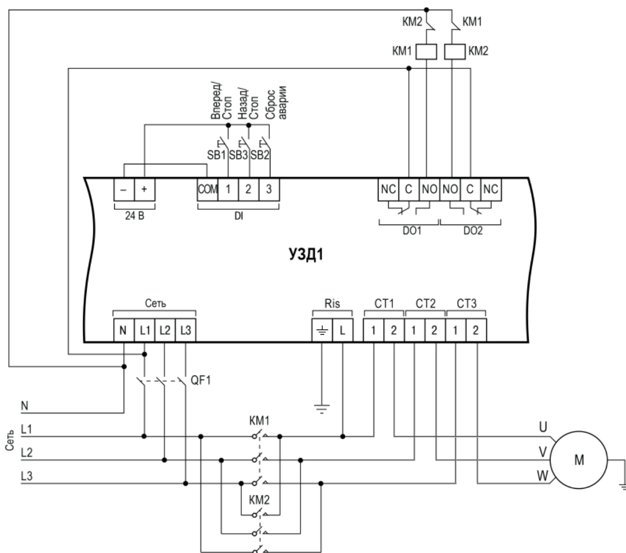
Рисунок 5.3 – Электрическая схема реализации реверсивного режима работы электродвигателя
